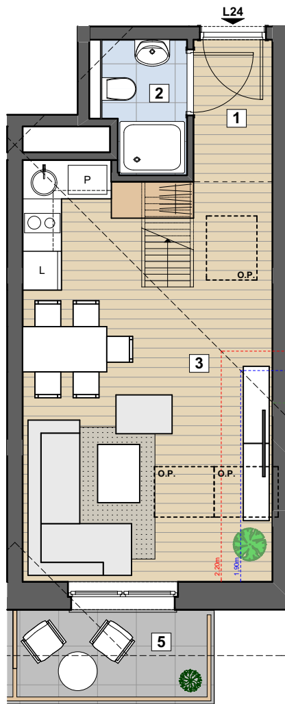
POZIOM_1
